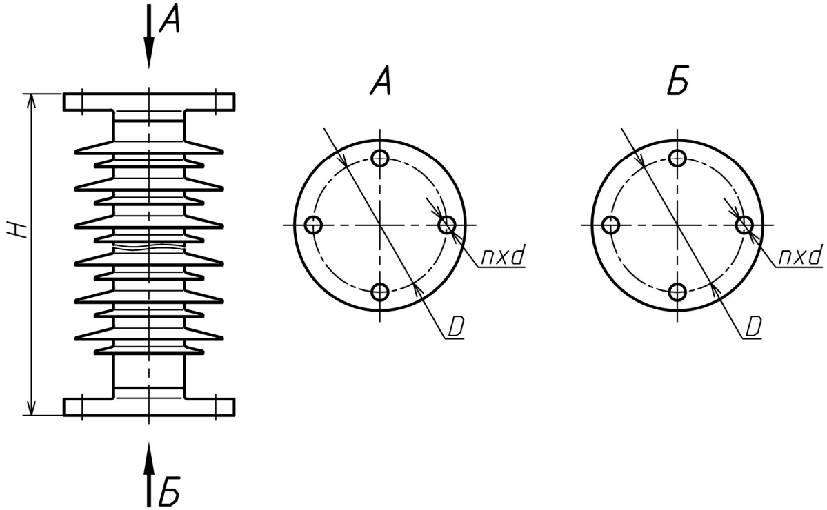
Присоединительные и габаритные размеры оконцевателей
