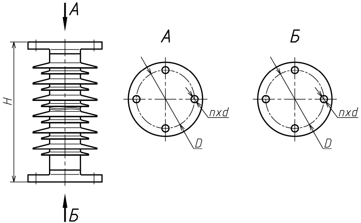
Присоединительные и габаритные размеры оконцевателей
