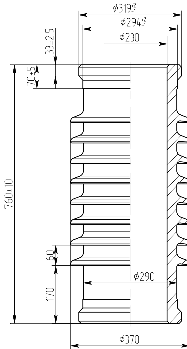
П760/230 УХЛ 1 чертёж АТКИ.686174.020 креслення
