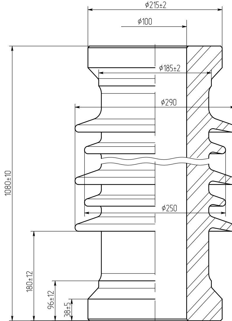
ППН - 1080/100 О чертёж НИЮД.757523.072 креслення
