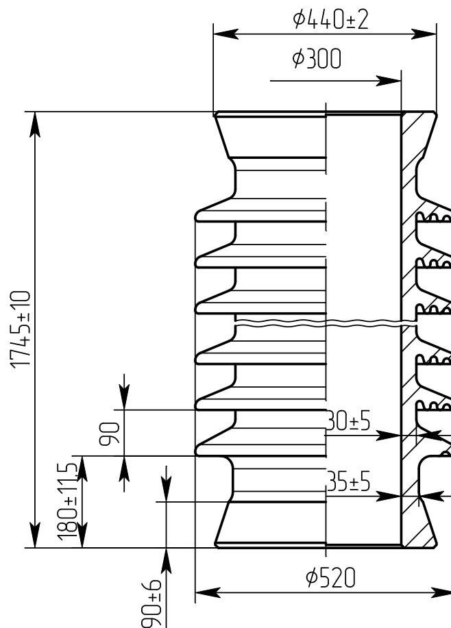
П 1745/300 У чертёж ИНЯЖ.757524.020 креслення
