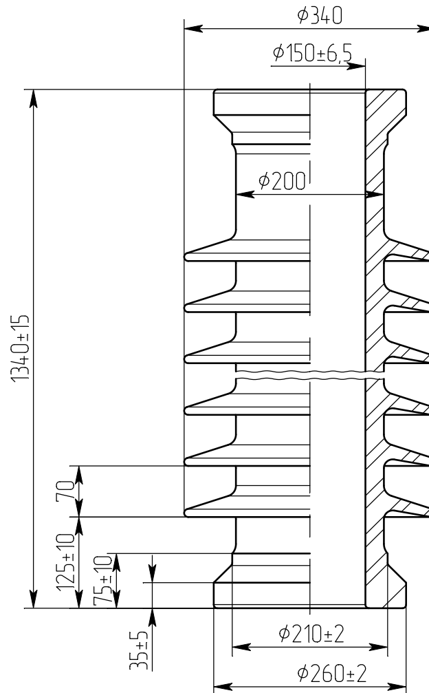
П 1340/150 О чертёж ИМЖК.757523.175 креслення
