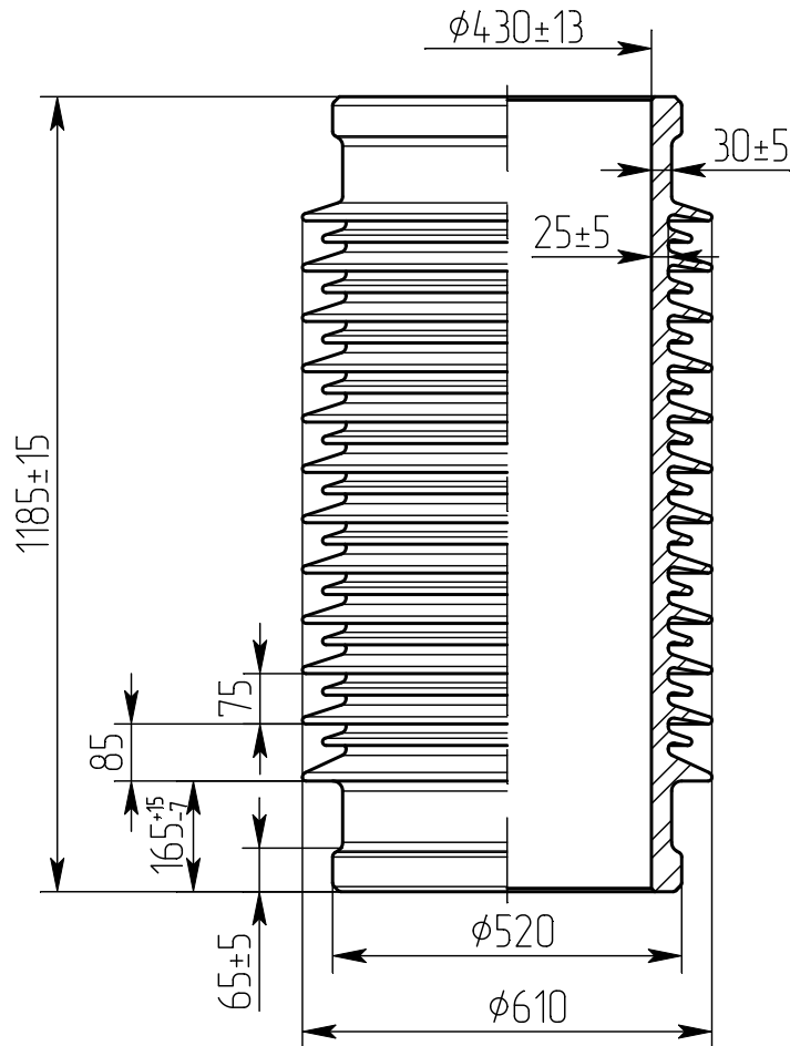
П 1185/430 О чертёж ИНЯЖ.757524.054 креслення
