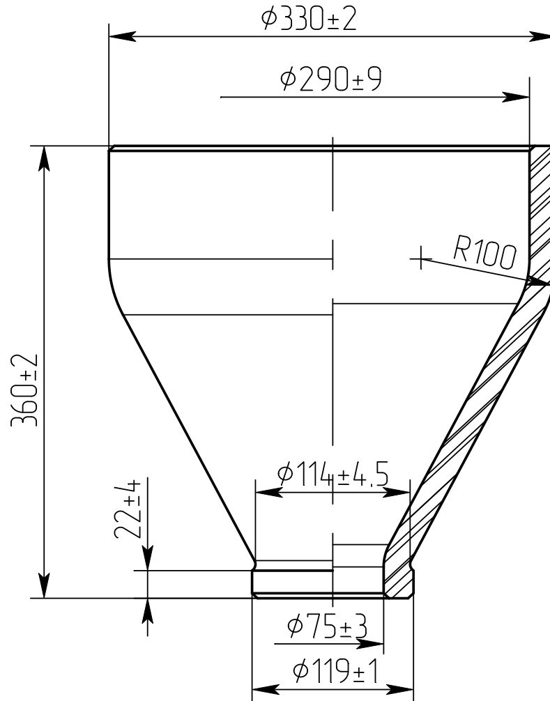
П 360/290 – 1 Г чертёж НИЮД.757513.030 креслення
